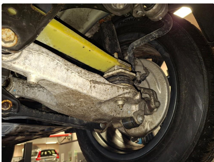
1.7 Kontrollert hjuloppheng
