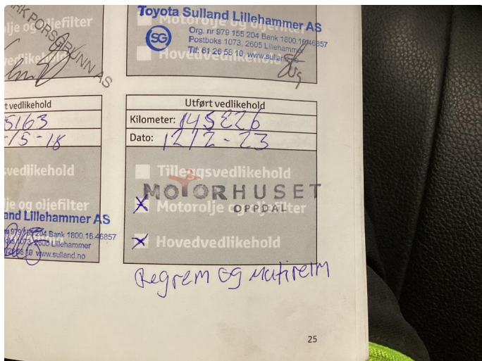
2.2 Registerreim/kjede
