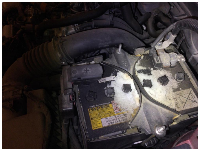
3.1 Startbatteri - svakt/defekt
