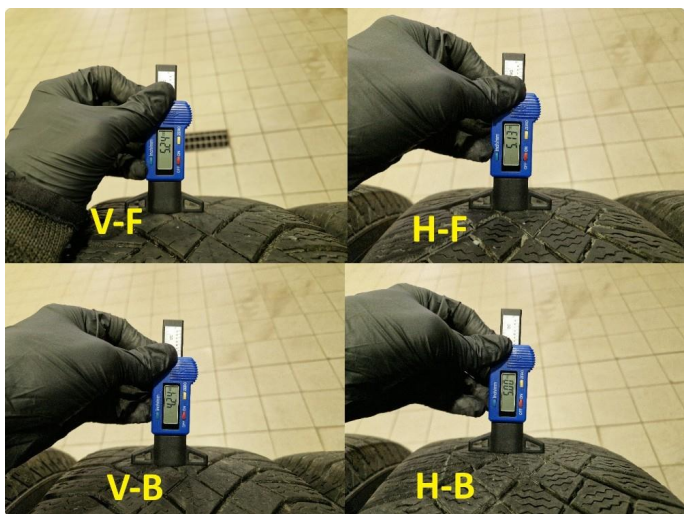
1.7 Dekkdybdemåling vinterdekk utført 18.08.2026 på km : 246.666
