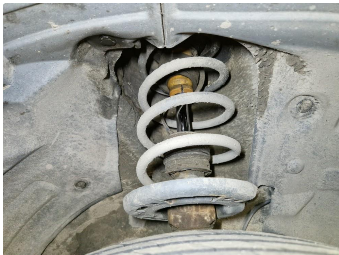
4.1 Sprukket støtdempermansjett h+v side fram.
