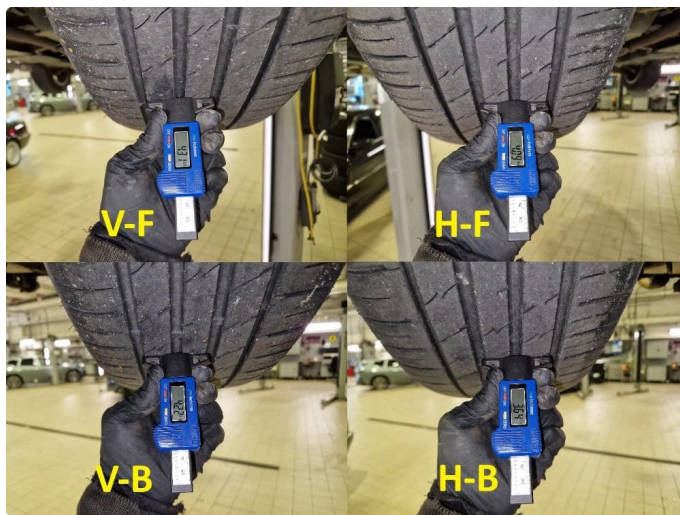
1.6 Dekkdybdemåling sommerdekk utført 18.08.2026 på km : 246.666
