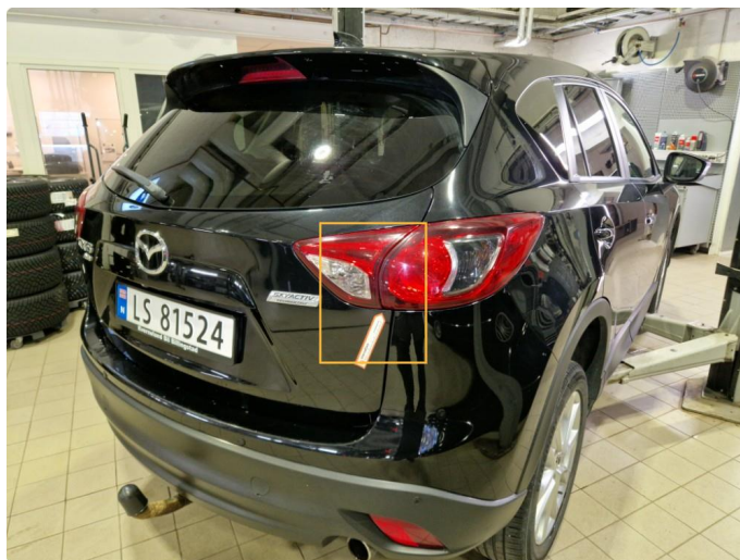
2.2 Sprekkdannelser indre + ytre baklykt h-side.
