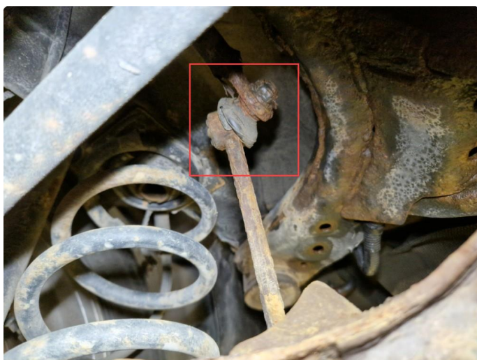
4.4 Utslitt / avgått lenkearm v-bak, defekt mansjett lenkearm h side bak.
