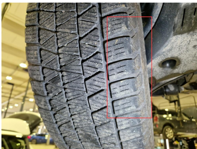
2.2 Noe skjeivslitasje innside vinterdekk h+v bak. 4-hjuls kontroll tatt etter takst.
