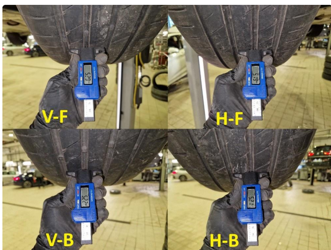
2.3 Mønsterdybde sommerdekk målt ved takst 23.05.2025, 43.902km.
