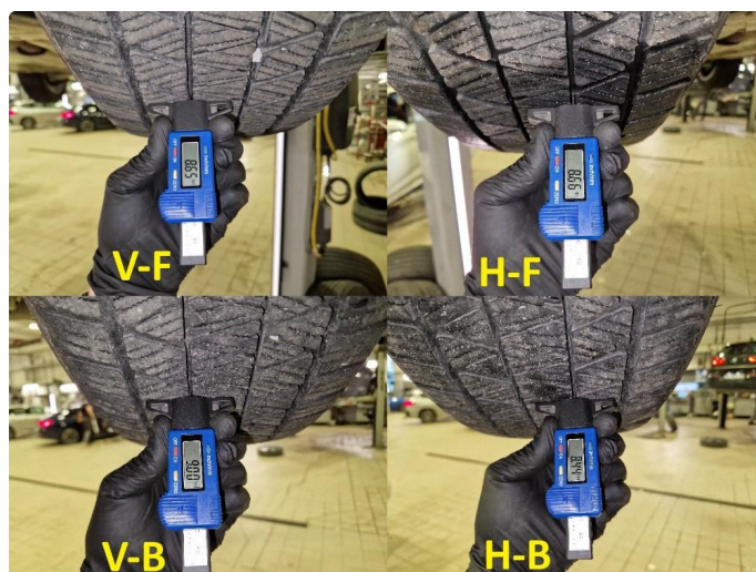
2.4 Mønsterdybde vinterdekk målt ved takst 23.05.2025, 43.902km.
