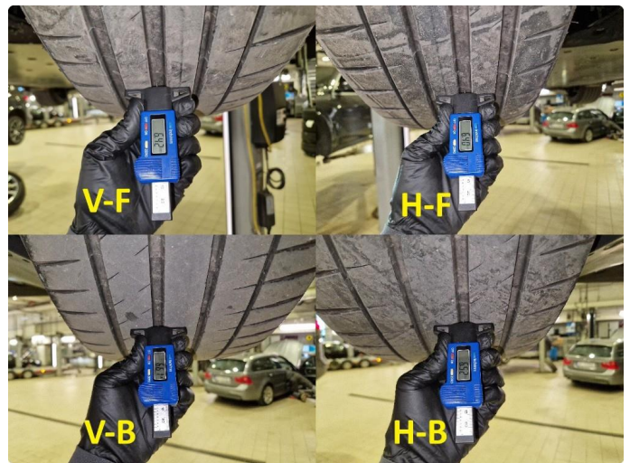
1.2 Dekkdybdemåling sommerdekk utført 19.05.2026 på km : 59.208.
