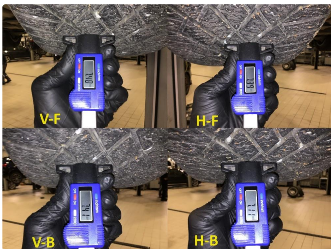
1.3 Mønsterdybde vinterdekk målt ved takst 13.05.24, 32.567km.
