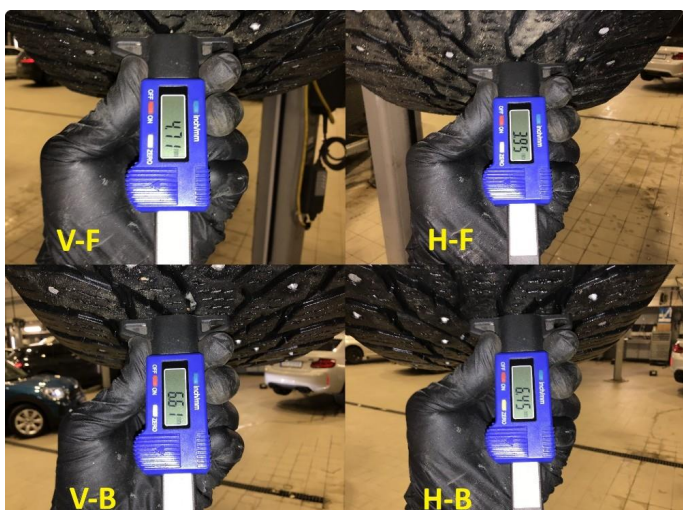
1.3 Mønsterdybde vinterdekk målt ved takst 21.02.2025, 108.137km. Nye dekk påsatt etter takst.
