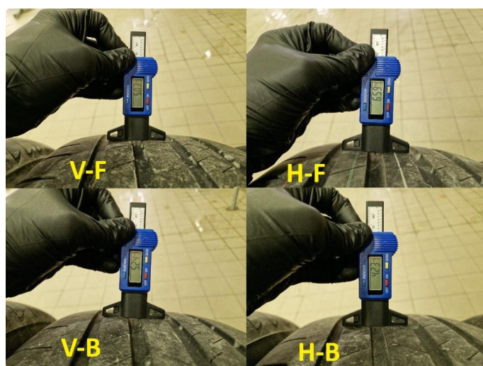
1.3 Mønsetrdybde sommerdekk målt ved innlevering, 62.935km.
