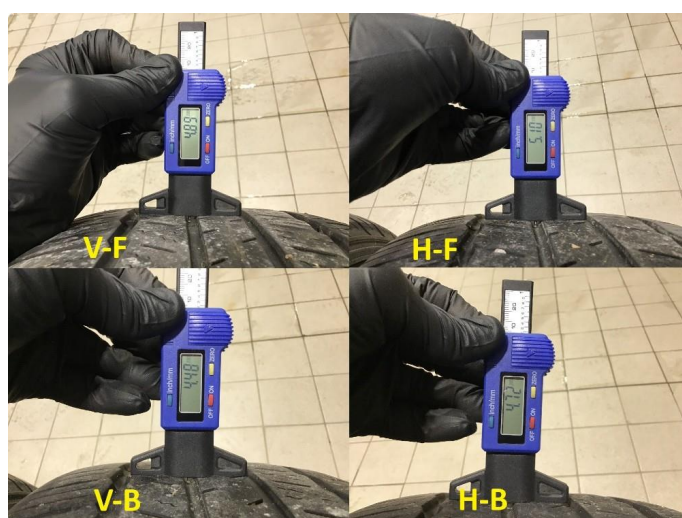
1.9 Dekkdybdemåling sommerdekk.
