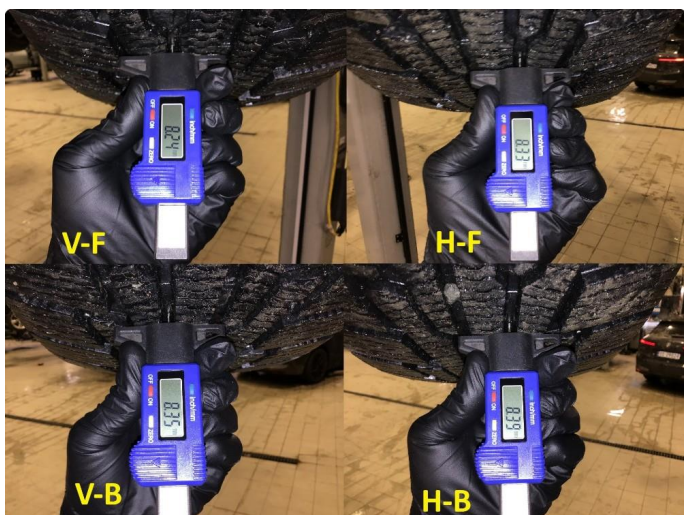
1.10 Dekkdybdemåling vinterdekk.
