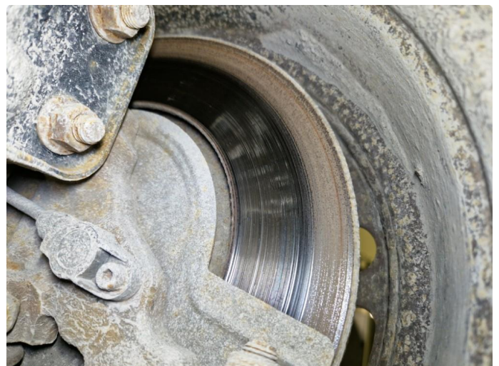
5.1 Noe slitasje bremsekiver fram, bremseklosser målt til 4,5mm.
