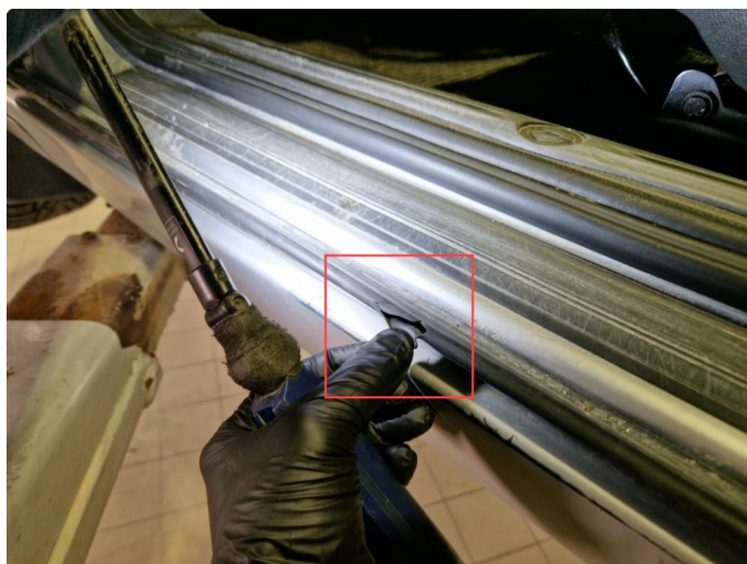
1.12 Skadet dørkarmlist v-fram.
