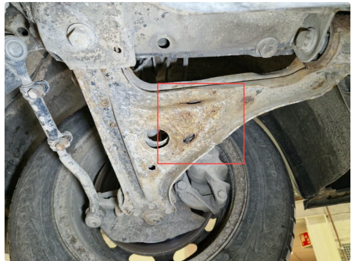
4.2 Rustdannelser / gjennomrustet bærebri v-side fram.
