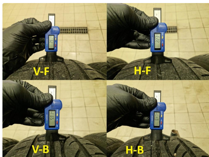
1.9 Dekkdybdemåling sommerdekk utført 17.04.2026 på km : 135.021
