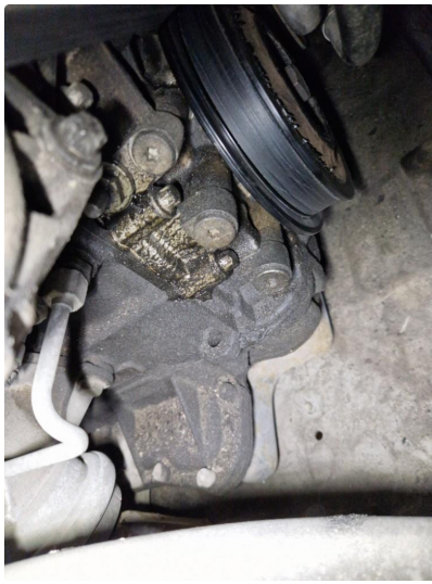
3.1 Oljelekkasjer motor.
