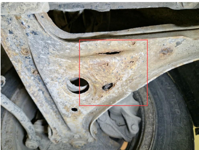
4.2 Rustdannelser / gjennomrustet bærebri v-side fram.
