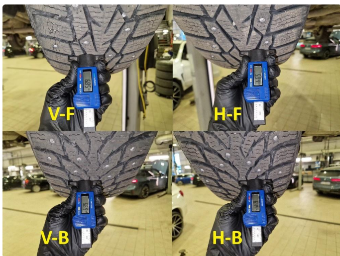
1.10 Dekkdybdemåling vinterdekk utført 17.04.2026 på km : 135.021
