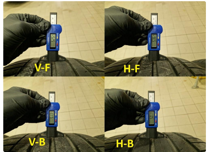
1.3 Dekkdybdemåling sommerdekk utført 04.02.2026
