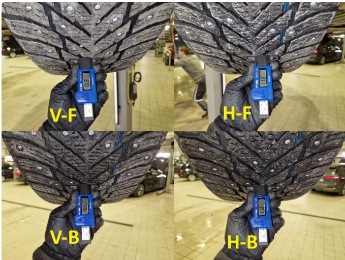
1.2 Dekkdybdemåling vinterdekk utført 26.11.2025 på km : 129.524
