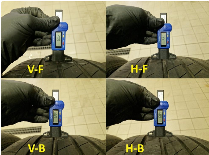
1.1 Mønsterdybde sommerdekk målt ved takst 20.05.2025, 20.878km.
