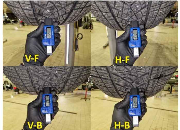
1.2 Mønsterdybde vinterdekk målt ved takst 20.05.2025, 20.878km.
