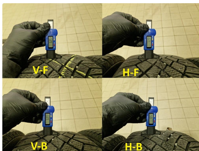
1.3 Mønsterdybde vinterdekk målt ved takst 28.08.2025, 25.824km.
