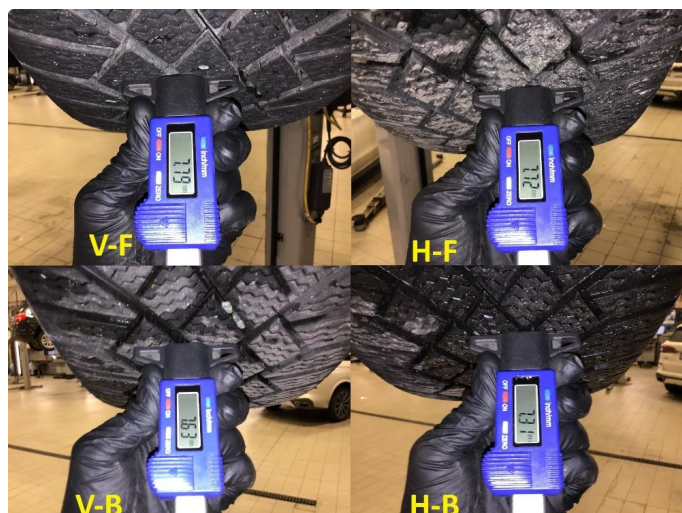
1.3 Mønsterdybde vinterdekk målt ved takst 24.10.2024, 27.729km.
