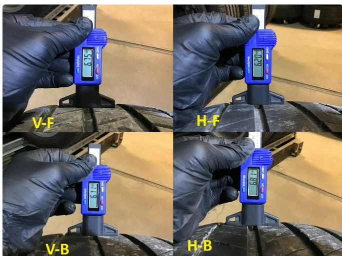
1.2 Mønsterdybde sommerdekk målt ved takst 24.10.2024, 27.729km.
