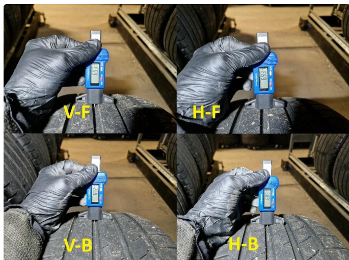
1.2 Dekkdybdemåling sommerdekk utført 26.03.2026 på km : 11.409
