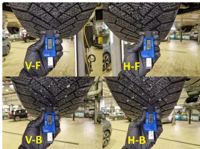
1.3 Dekkdybdemåling vinterdekk utført 26.03.2026 på km : 11.409
