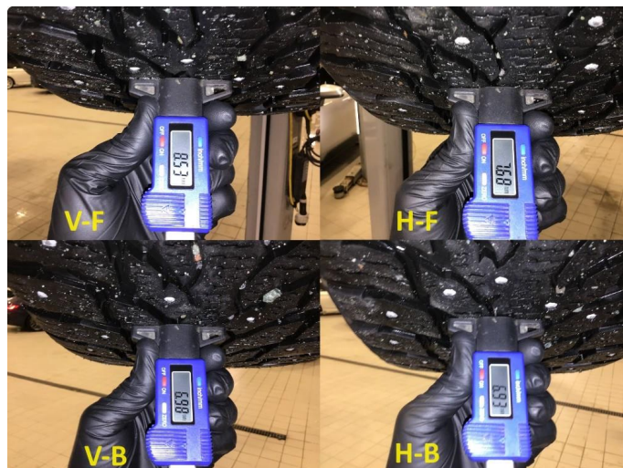
1.5 Mønsterdybde vinterdekk målt ved takst 23.01.24, 114.228km. Nye dekk påsatt etter takst.
