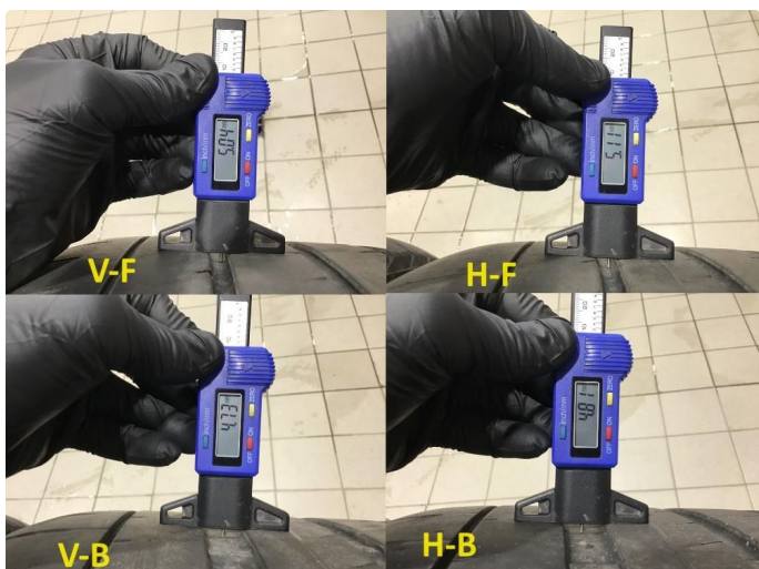
1.4 Mønsterdybde sommerdekk målt ved takst 23.01.24, 114.228km.
