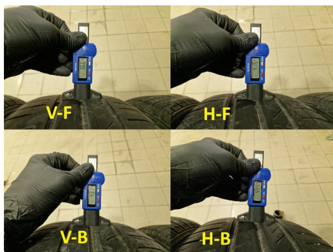
2.13 Dekkdybdemåling sommerdekk utført 26.01.2026 på km : 116.555.
