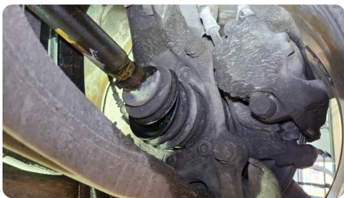
4.1 Drivakselledd defekt Mansjetter defekt, liten ulyd i akselledd
