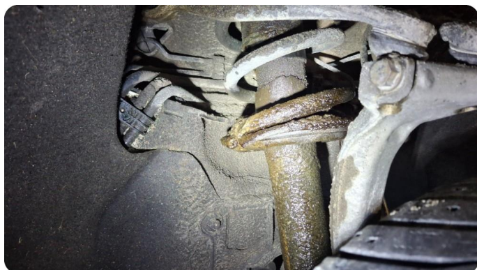
3.1 Støtdemper lekkasje
