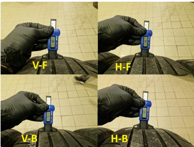
1.3 Mønsterdybde sommerdekk målt ved takst 31.10.2025, 32.153km.
