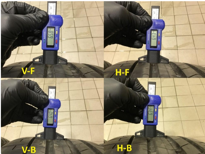
1.1 Mønsterdybde sommerdekk målt ved takst 23.01.2025, 4.931km.
