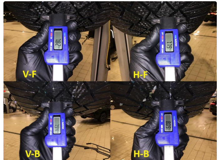
1.2 Mønsterdybde vinterdekk målt ved takst 23.01.2025, 4.931km.
