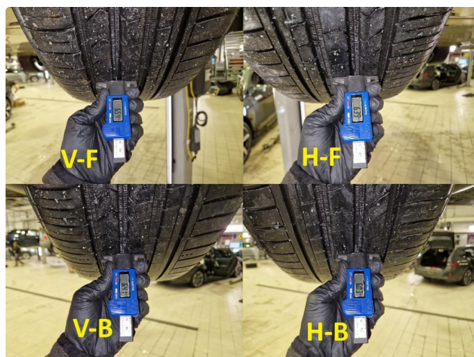
1.3 Dekkdybdemåling sommerdekk utført 24.11.2025 på km : 101.667
