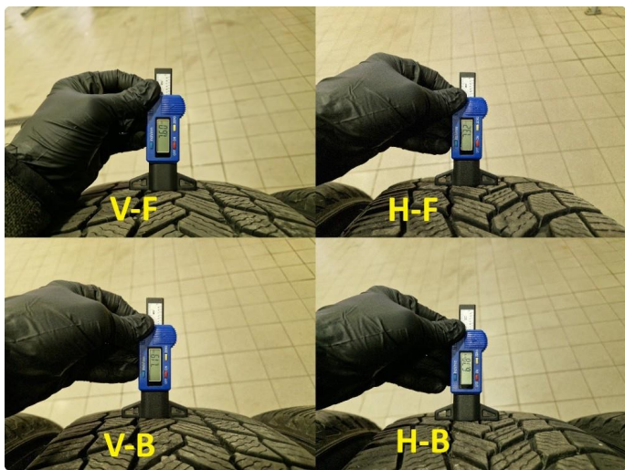
1.4 Dekkdybdemåling vinterdekk utført 24.11.2025 på km : 101.667
