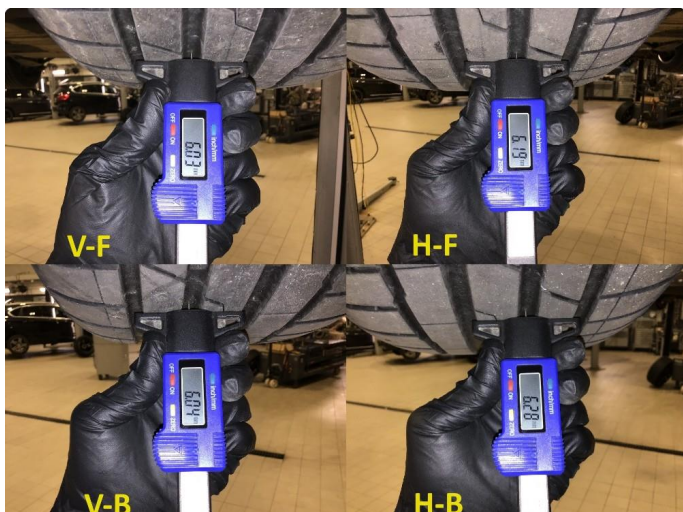
1.1 Mønsterdybde sommerdekk målt ved takst 18.07.2024, 29.857km.
