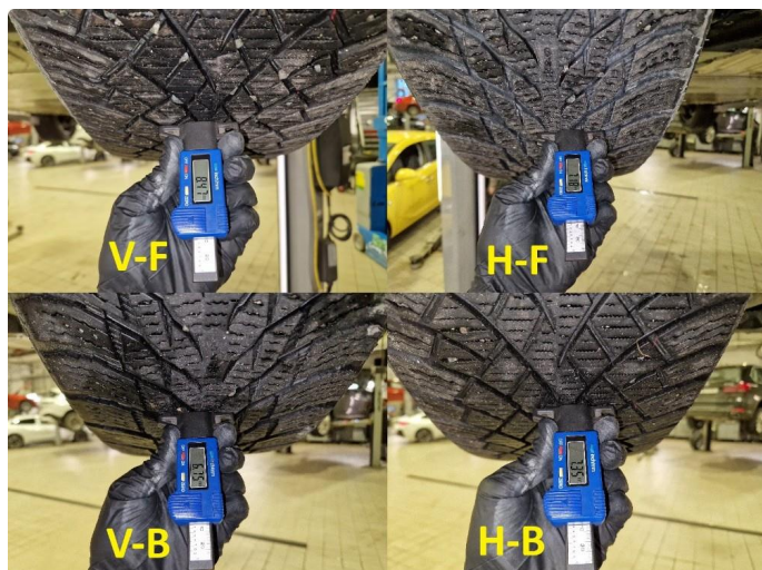
1.1 Dekkdybdemåling vinterdekk utført 06.11.2025 på km : 51.750
