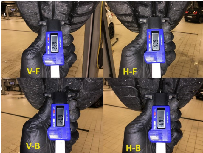
1.2 Mønsterdybde sommerdekk , målt ved takst 28.06.24 , 14150km.
