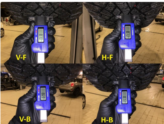
1.3 Mønsterdybde vinterdekk målt ved takst 03.02.2025.
