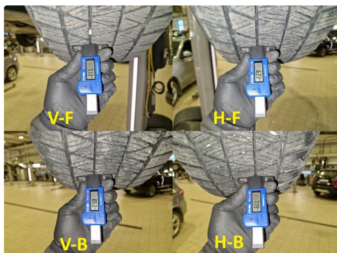
1.2 Mønsterdybde sommerdekk målt ved takst 23.05.2025, 50.079km. 2 nye dekk påsatt etter takst.
