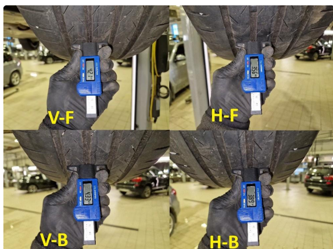
1.1 Mønsterdybde sommerdekk målt ved takst 23.05.2025, 50.079km.
