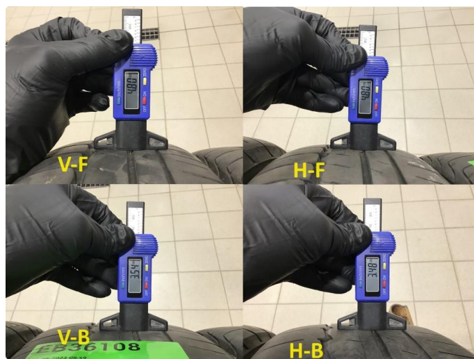
1.3 Mønsterdybde sommerdekk målt ved takst 25.03.24, 75.968km.
