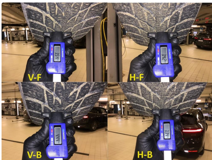
1.4 Mønsterdybde vinterdekk målt ved takst 25.03.24, 75.968km. Nye dekk påsatt etter takst.
