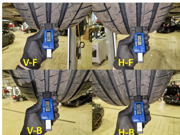
1.2 Dekkdybdemåling sommerdekk utført 11.06.2025 på km : 106871
