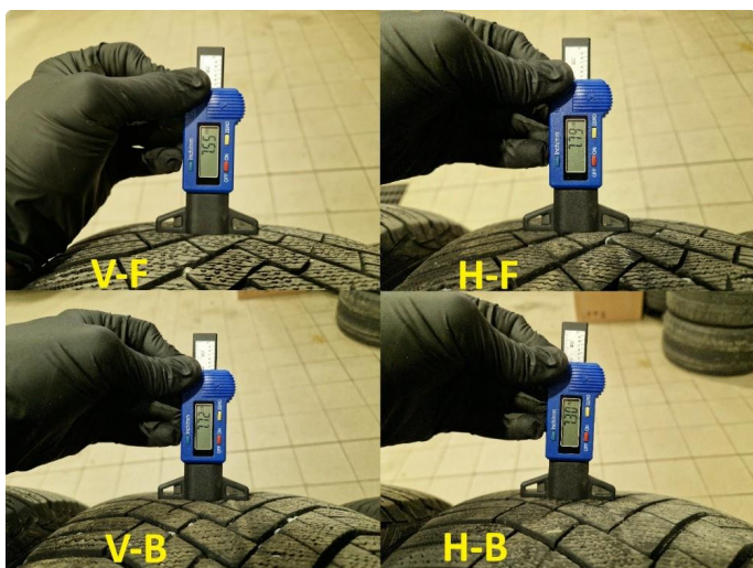
1.3 Dekkdybdemåling vinterdekk utført 11.06.2025 på km : 106871
