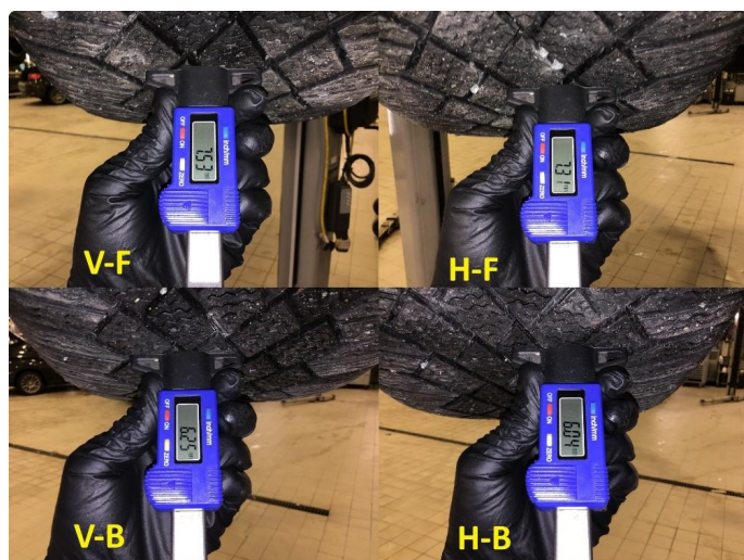
1.3 Mønsterdybde vinterdekk målt ved takst 15.01.2025, 44.897km.
