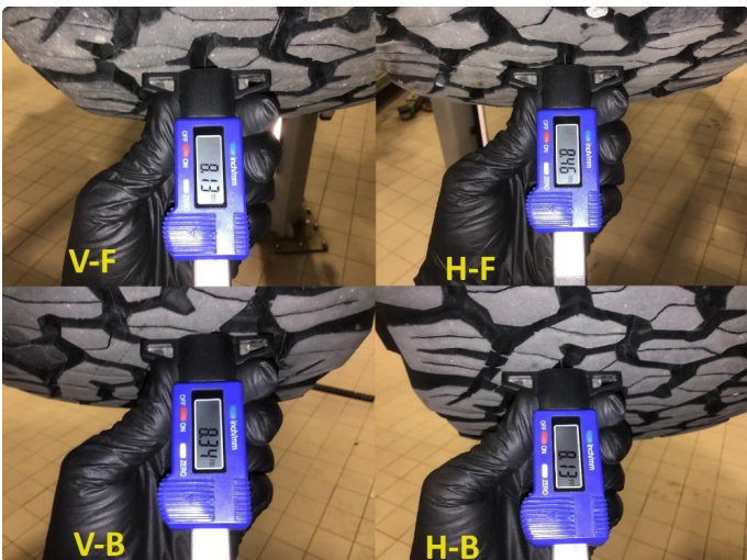
1.3 Dekkdybdemåling sommerdekk utført 07.06.2024 på km : 72211 .
