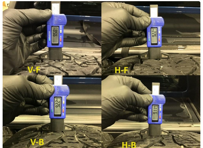
1.4 Dekkdybdemåling vinterdekk utført 07.06.2024 på km : 72211 .
