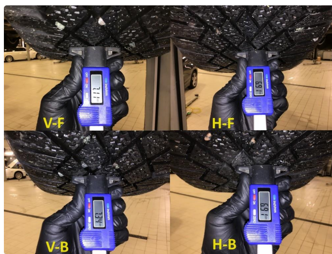
1.4 Mønsterdybde vinterdekk målt ved takst 23.01.24, 30.729km.
