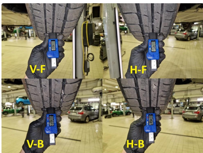
1.4 Dekkdybdemåling sommerdekk , måling utført 29.08.2025 på km : 36560.
