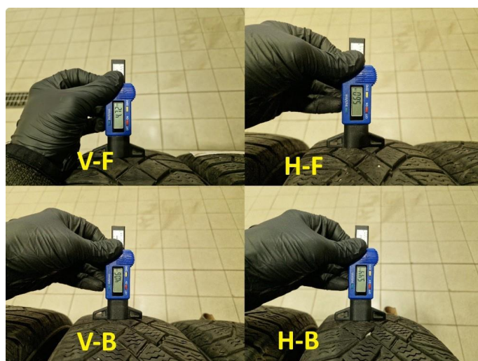
1.5 Dekkdybdemåling vinterdekk , måling utført 29.08.2025 på km : 36560.
