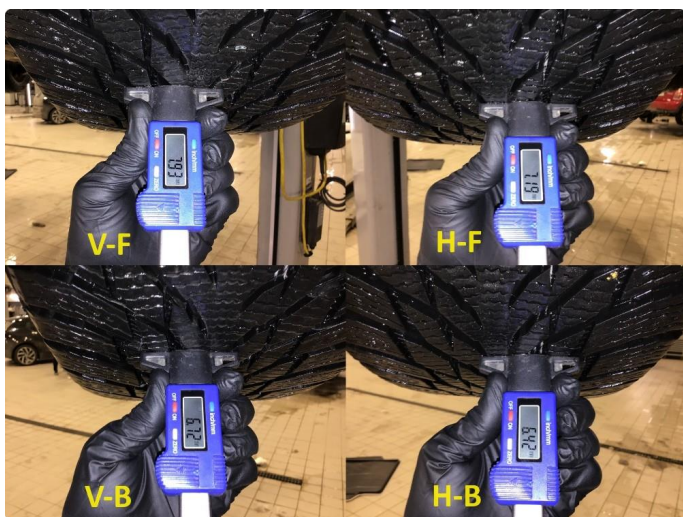
1.3 Mønsterdybde vinterdekk målt ved takst 23.02.24, 34.009km.
