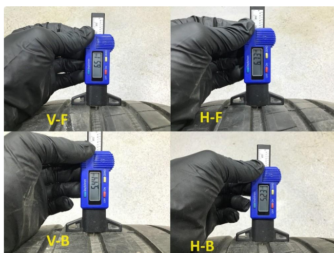
1.2 Mønsterdybde sommerdekk målt ved takst 23.02.24, 34.009km.
