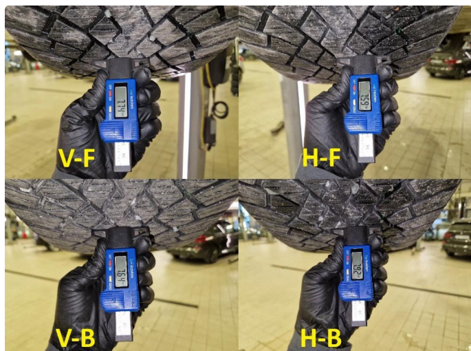
1.1 Mønsterdybde vinterdekk målt ved takst 18.06.2025, 25.299km.
