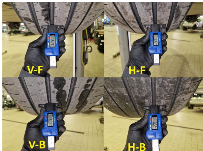
1.2 Sommerdekk målt ved mottak 19.06.2025, 28.382km.
