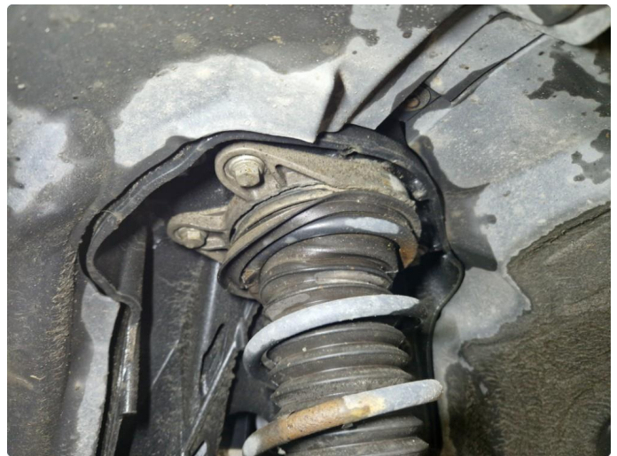
6.1 Fjærbeinslager slitt/defekt
