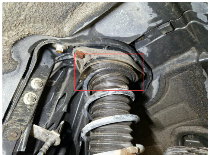
6.2 Støvmansjett defekt
