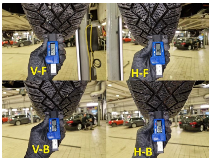
3.8 Mønsterdybde vinterdekk målt ved takst 23.10.2025, 175.261km.
