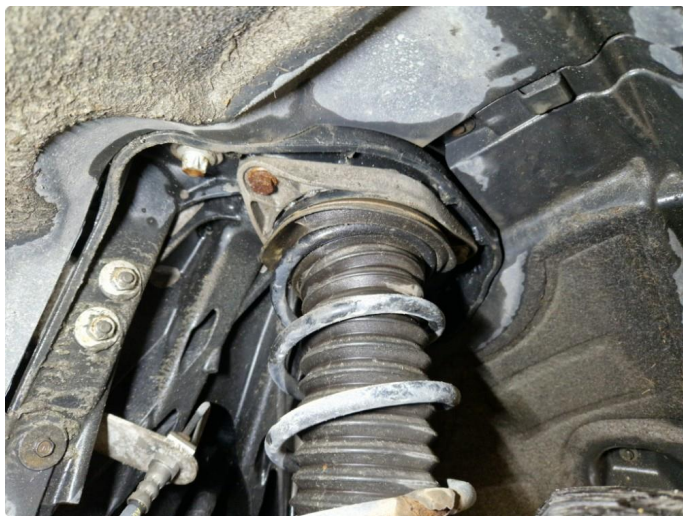
6.1 Fjærbeinslager slitt/defekt
