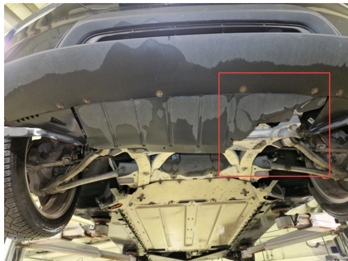
3.1 Skadet fremre midtre beskyttelsesplate.
