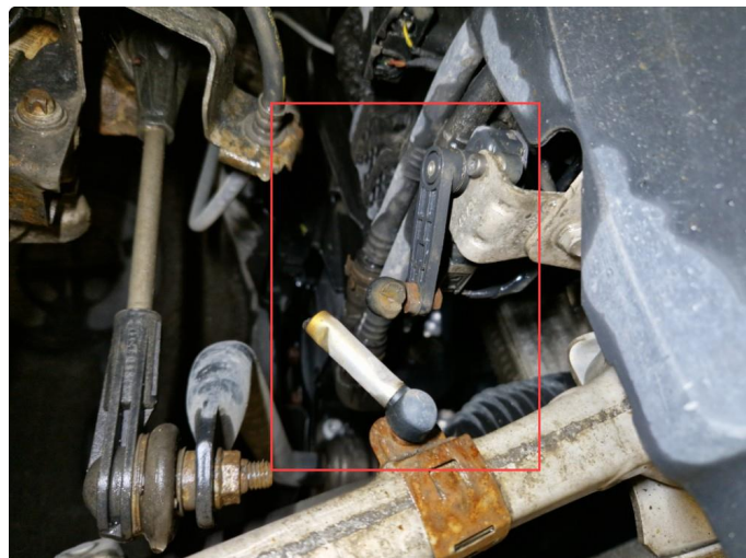
2.1 Skadet stag til nivåsensor v-fram.
