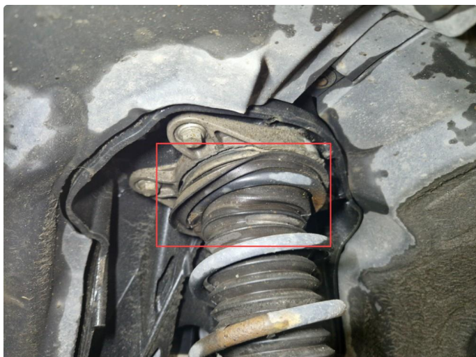
6.2 Støvmansjett defekt
