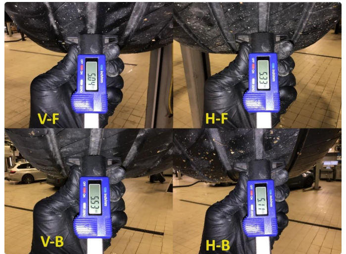
1.3 Mønsterdybde sommerdekk målt ved takst 27.08.2024, 44.262km.
