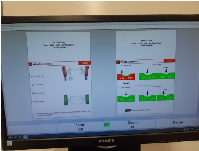
2.1 4-hjulsmåling/forstillingskontroll
