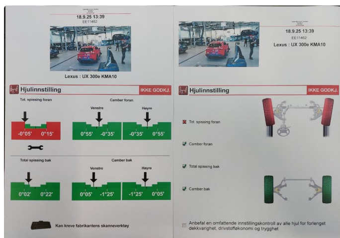
2.1 4-hjulsmåling/forstillingskontroll
