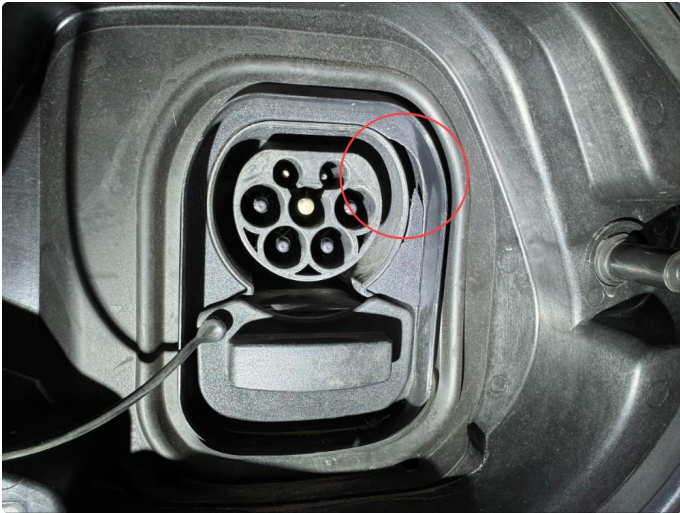
2.1 Ladekontakt skadet
