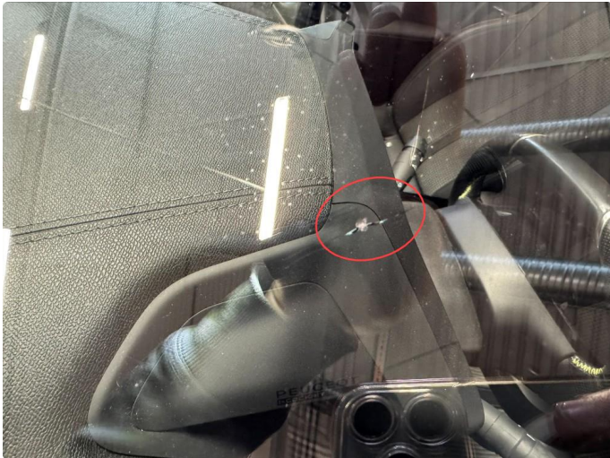
2.3 Steinsprang
